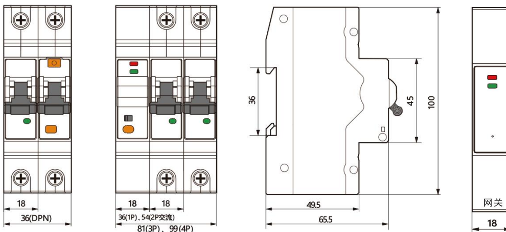
图3 断路器及网关尺寸
