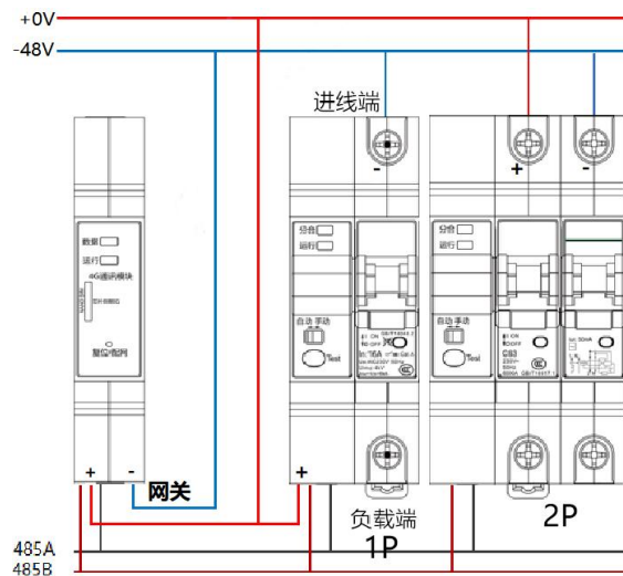
图 5 直流接线图
