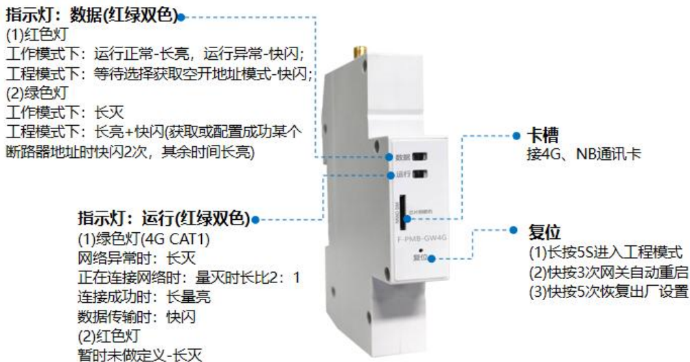
图2 网关面板说明
