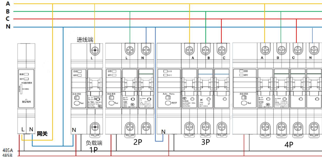
图 4 交流接线图
