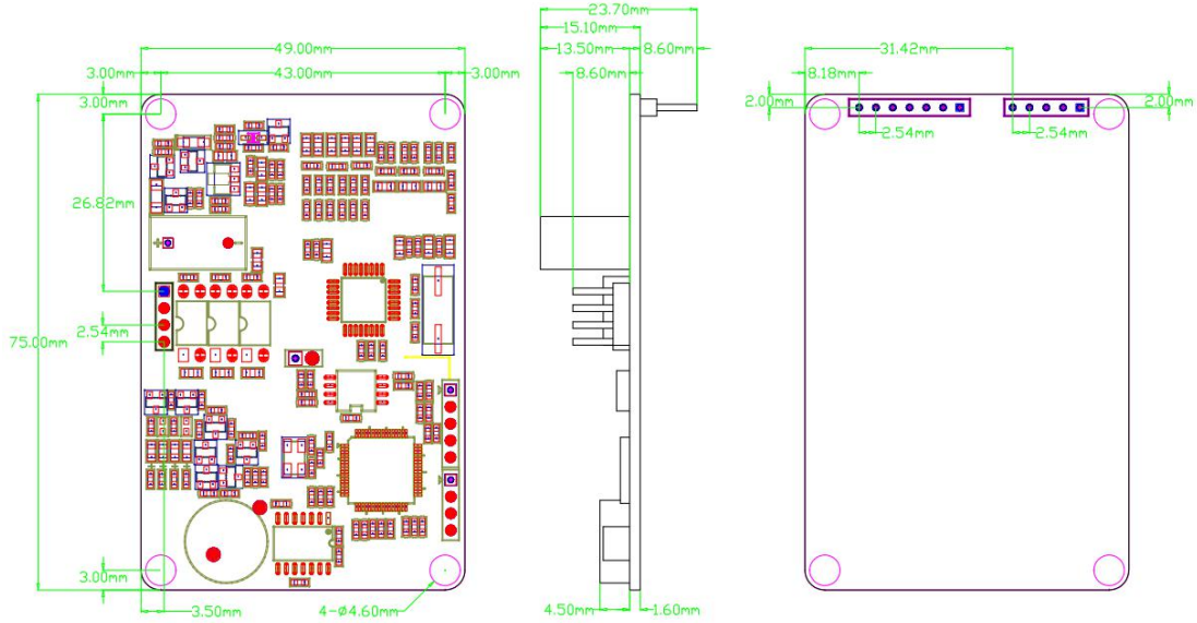
图 4-1 外形及安装尺寸图
