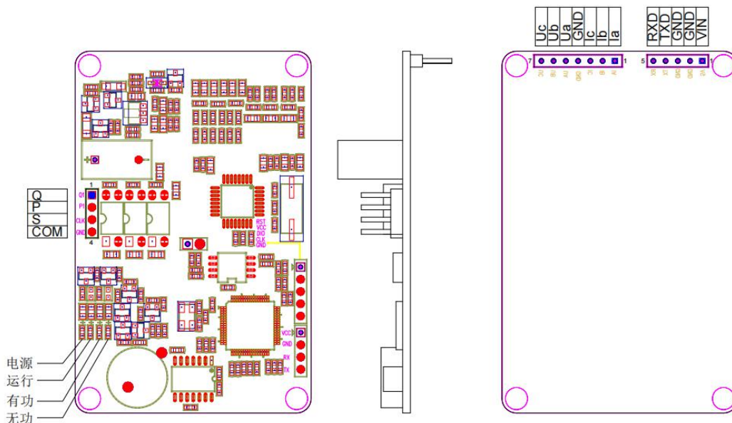
图 3-1 嵌入式 1 路模拟量线损模块指示灯位置及定义
