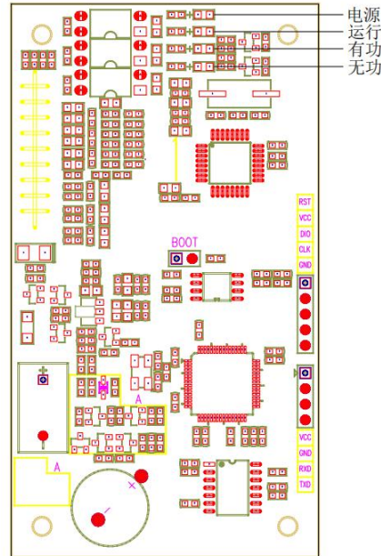
图 3-1 嵌入式 1 路模拟量线损模块指示灯位置及定义
