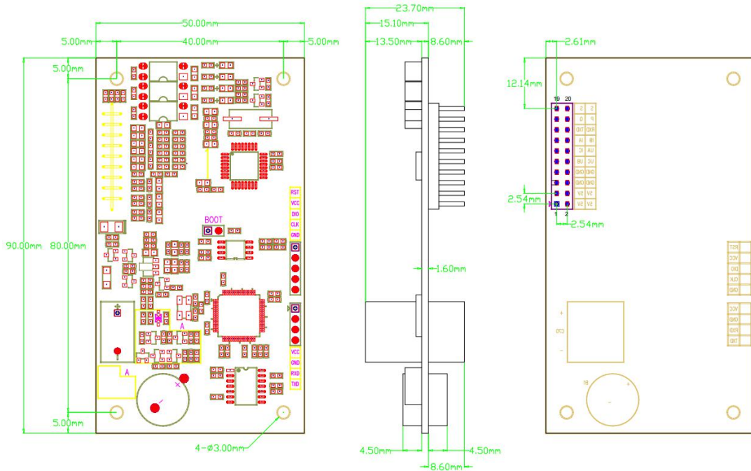
图 4-1 外形及安装尺寸图
