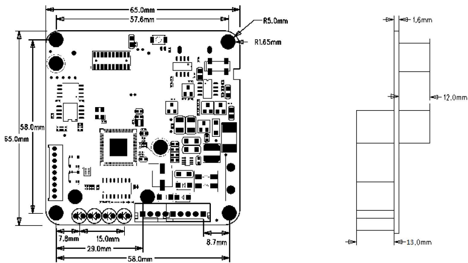
Router 尺寸
