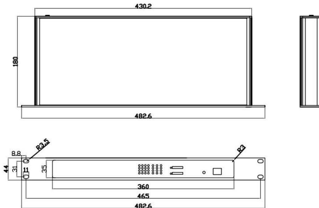
通信管理机尺寸
