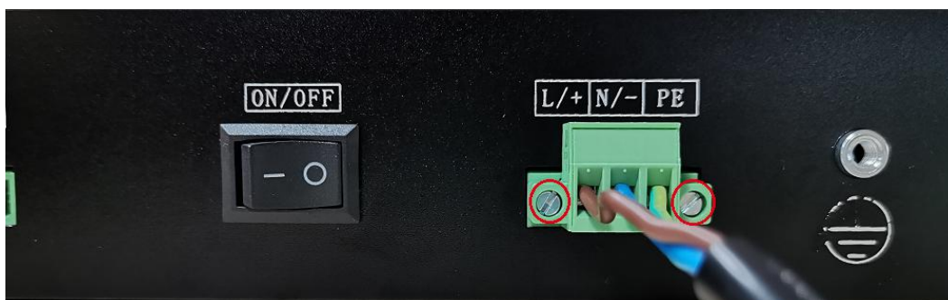
电源线接法
