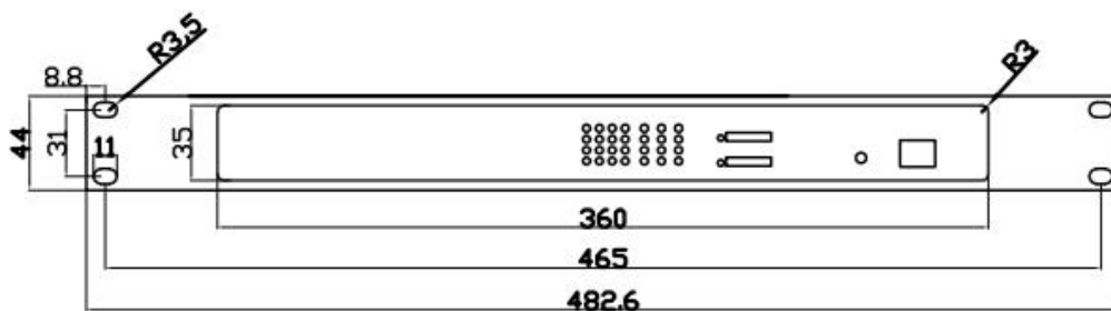
固定片尺寸
