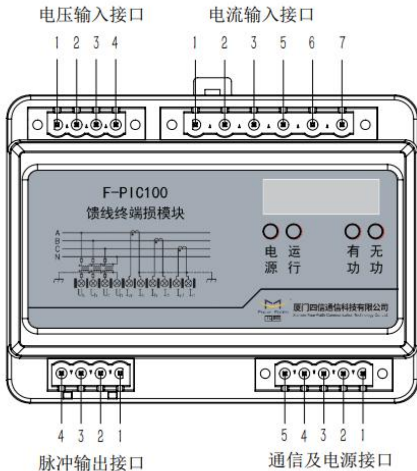
F-PIC100 端子接线示意图
