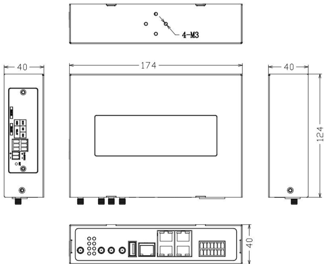
通信管理机尺寸
